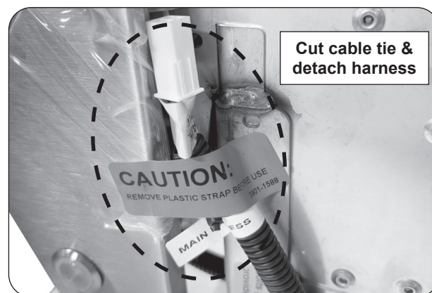
Fig. 26-2 Cut cable-tie
