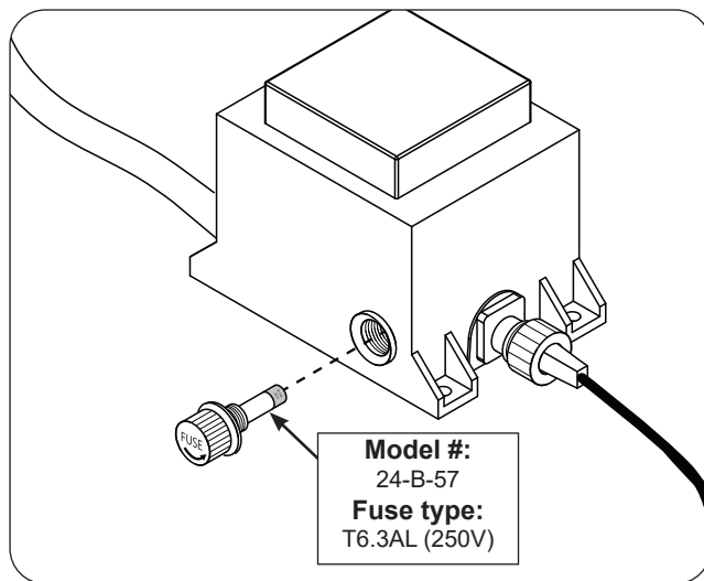
Fig. 43-1 Replace fuse
